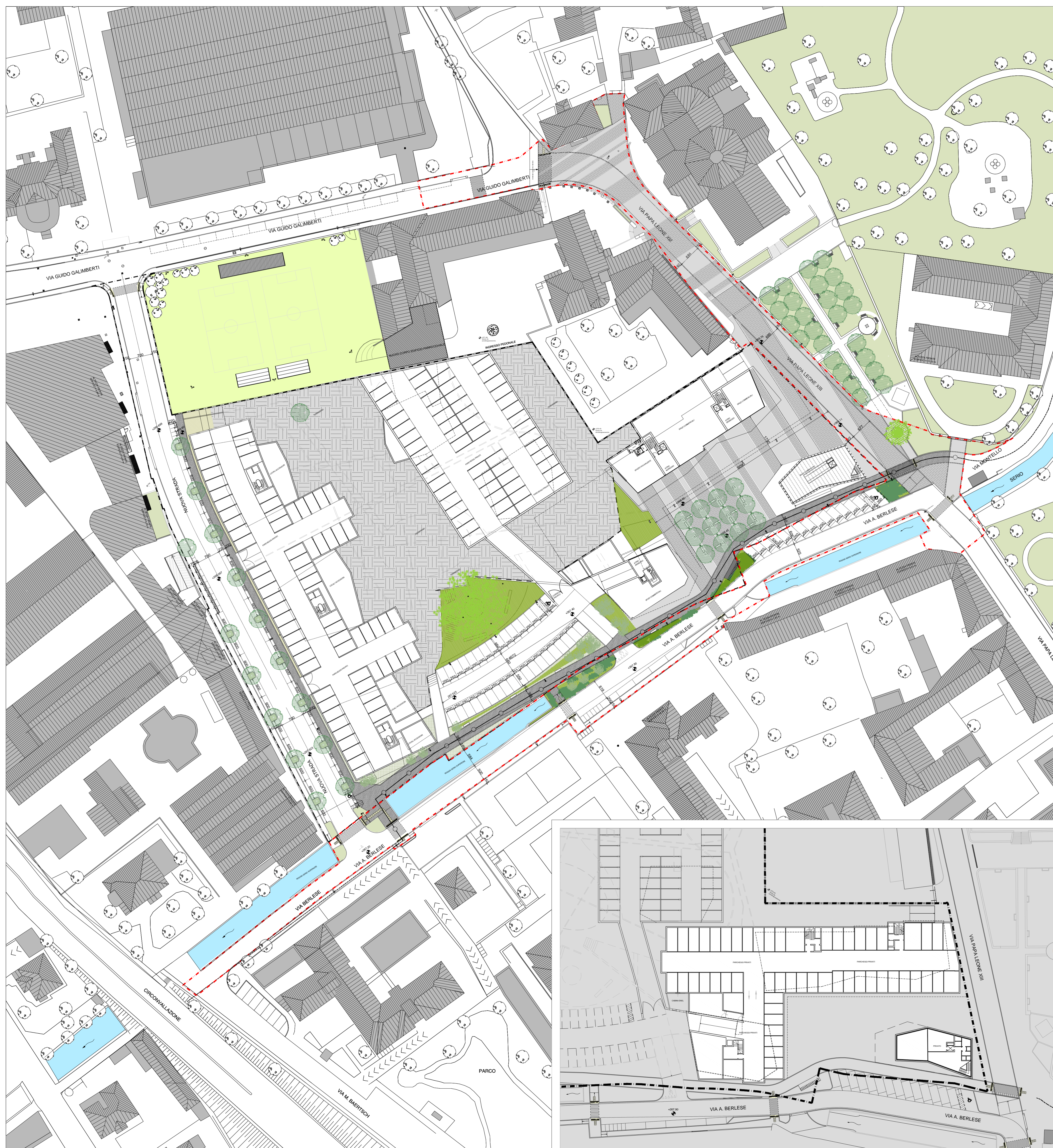
PLANIMETRIA - LIVELLO 0
