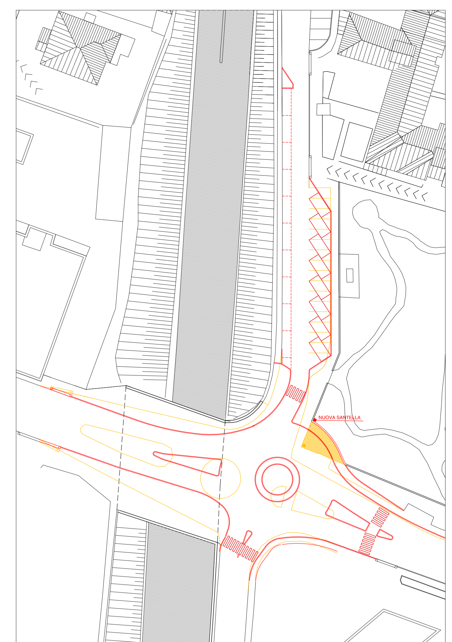
NUOVA ROTATORIA - SOVRAPPORZIONI - SCALA 1:500
