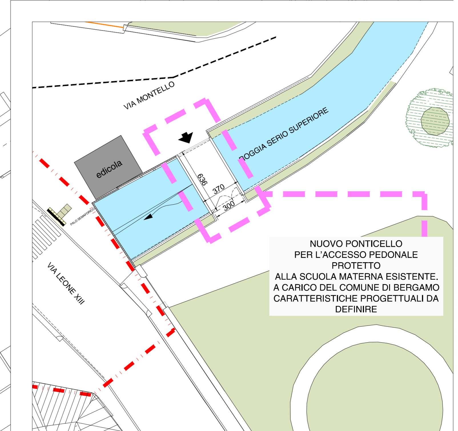
PONTECILLO PEDONALE SULLA ROGGIA SERIO - PLANIMETRIA - SCALA 1:200
