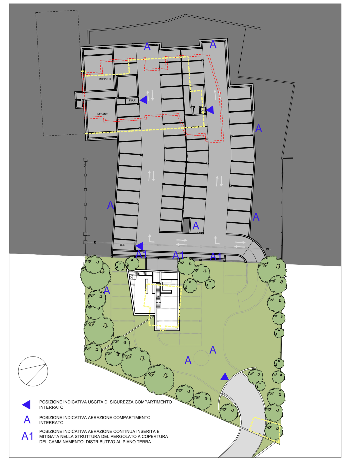
Planimetria livello interrato -1
