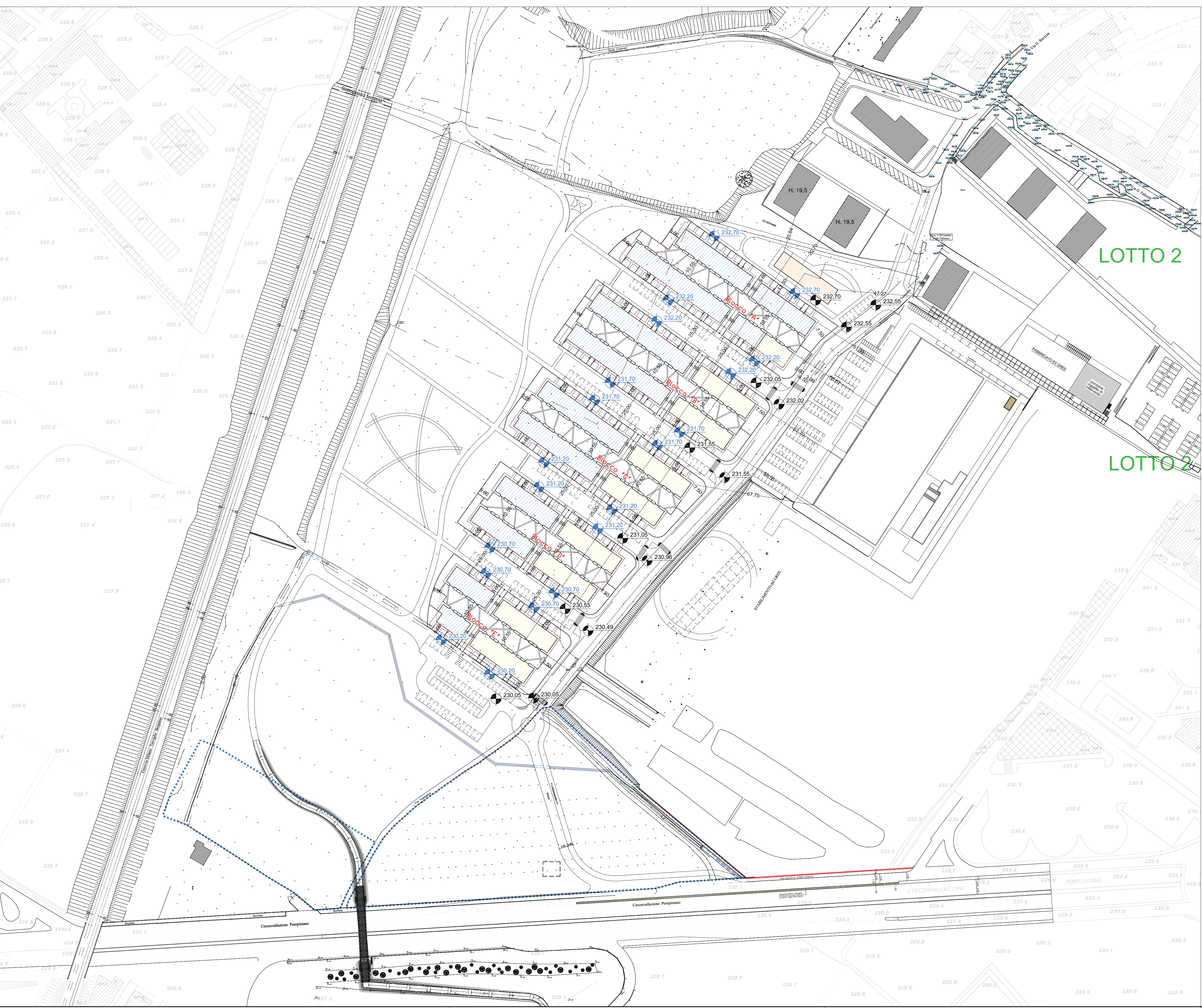
PLANIMETRIA GENERALE - scala 1:1000
