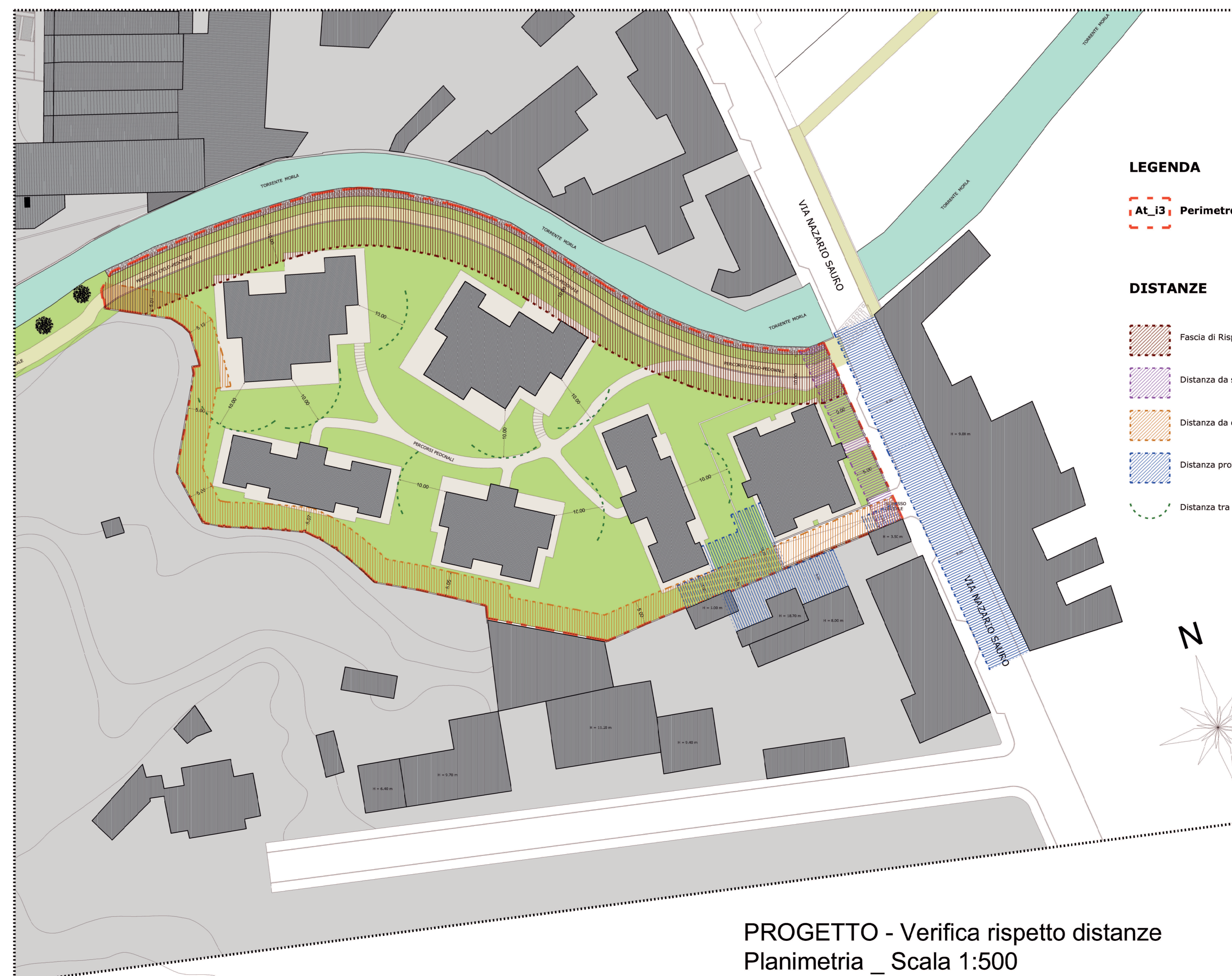
PROGETTO - Verifica Indice Permeabilità e Legge 122/89 Piano interrato _ Scala 1:500
