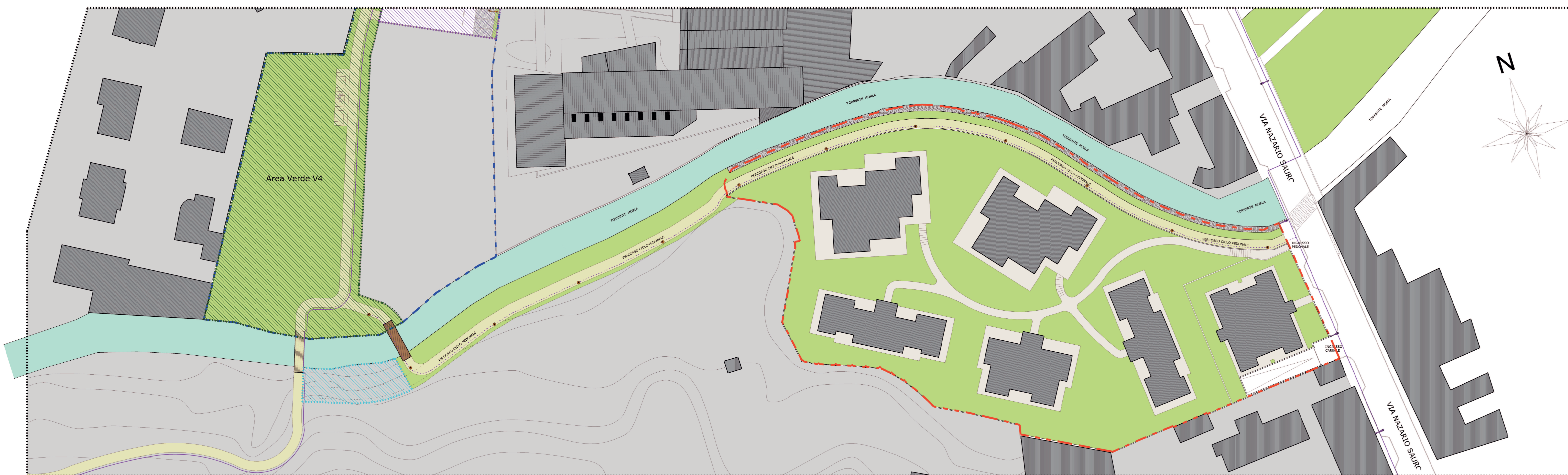
RETE PUBBLICA ILLUMINAZIONE Planimetria _ Scala 1:500
