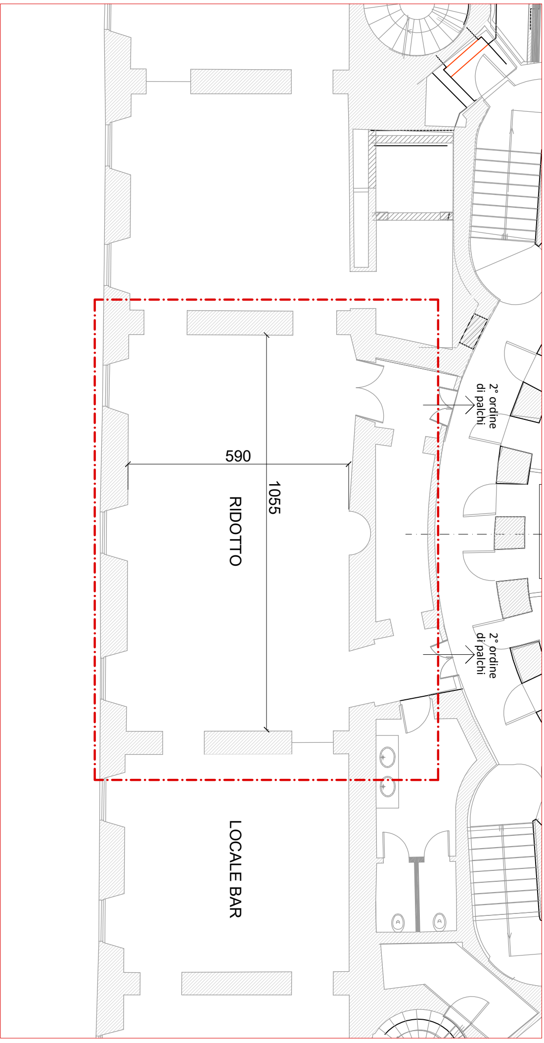
planimetria quota 2° ordine di palchi
